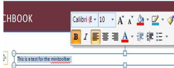
Fig 5.6 Mini Toolbar
