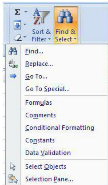
Fig. 4.31 Goto Function
