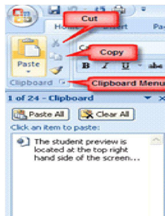
Fig 3.21 Clipboard button
