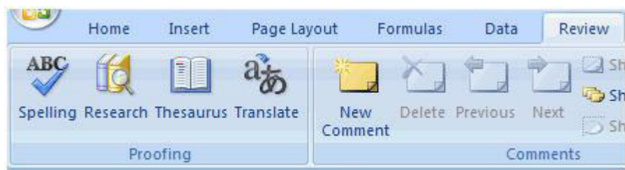
Fig. 4.32 Spell Check
